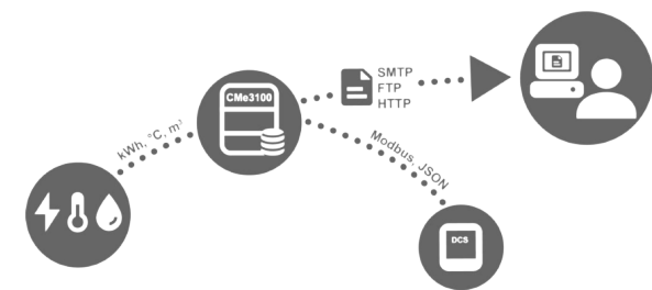
Abb. 1: Messdatenerfassung und Integration in SCADA-System
