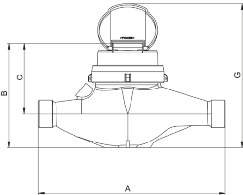
MTWcoder® MP mit Zählerdeckel
