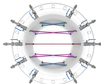
Nasse Sensoren angeordnet in fünf parallelen Ebenen
