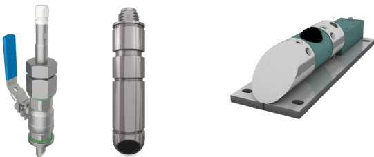
FT-S und FT-L Feedthrough-Sensoren und Innen montierter Sensor TD-IM
