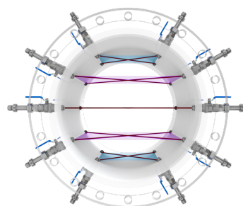
Capteurs mouillés disposés en cinq plans parallèles
