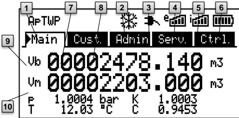
Fig. 24 Display layout
