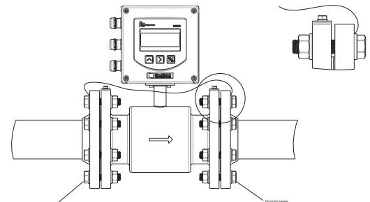
Abbildung 18: Potentialfreie Montage
