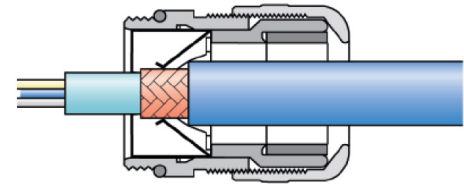
Abbildung 29: Kabeleinführung
