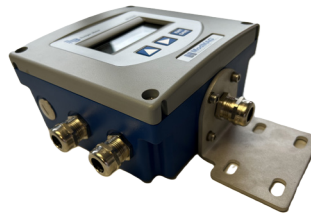
Abbildung 20: Zwei Schrauben herausdrehen
