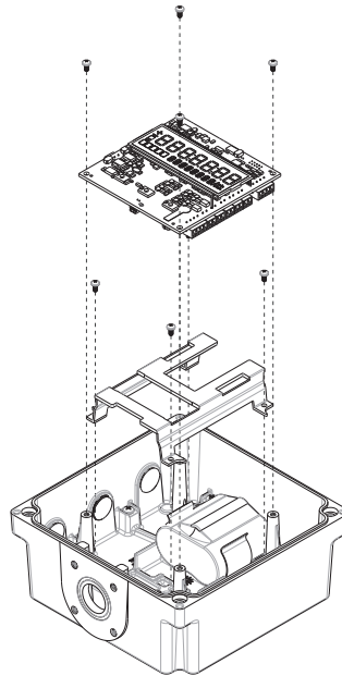
Abbildung 24: Komponenten des Verstärkergehäuses – Explosionszeichnung
