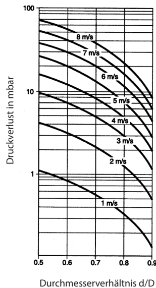
Abbildung 10: Druckverlustdiagramm
