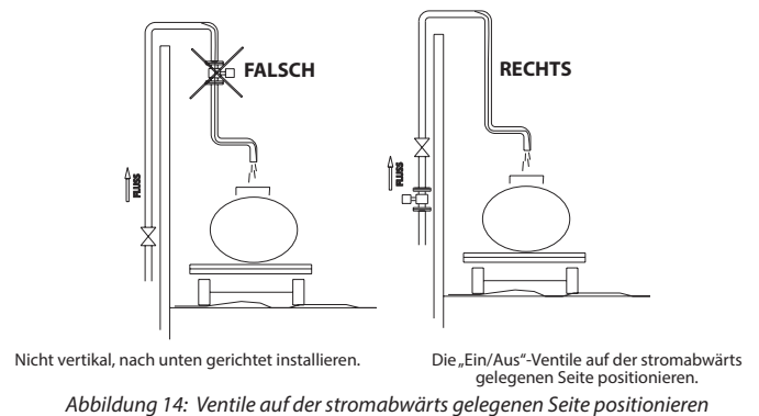
Abbildung 14: Ventile auf der stromabwärts gelegenen Seite positionieren
