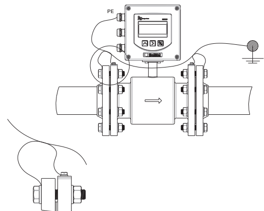
Abbildung 19: Erdung für elektrisch gestörte Umgebung
