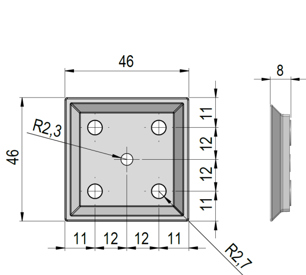
Abb. 10: Wandhalterung
