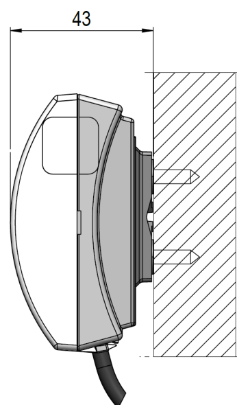
Abb. 11: Montiert auf Wandhalterung
