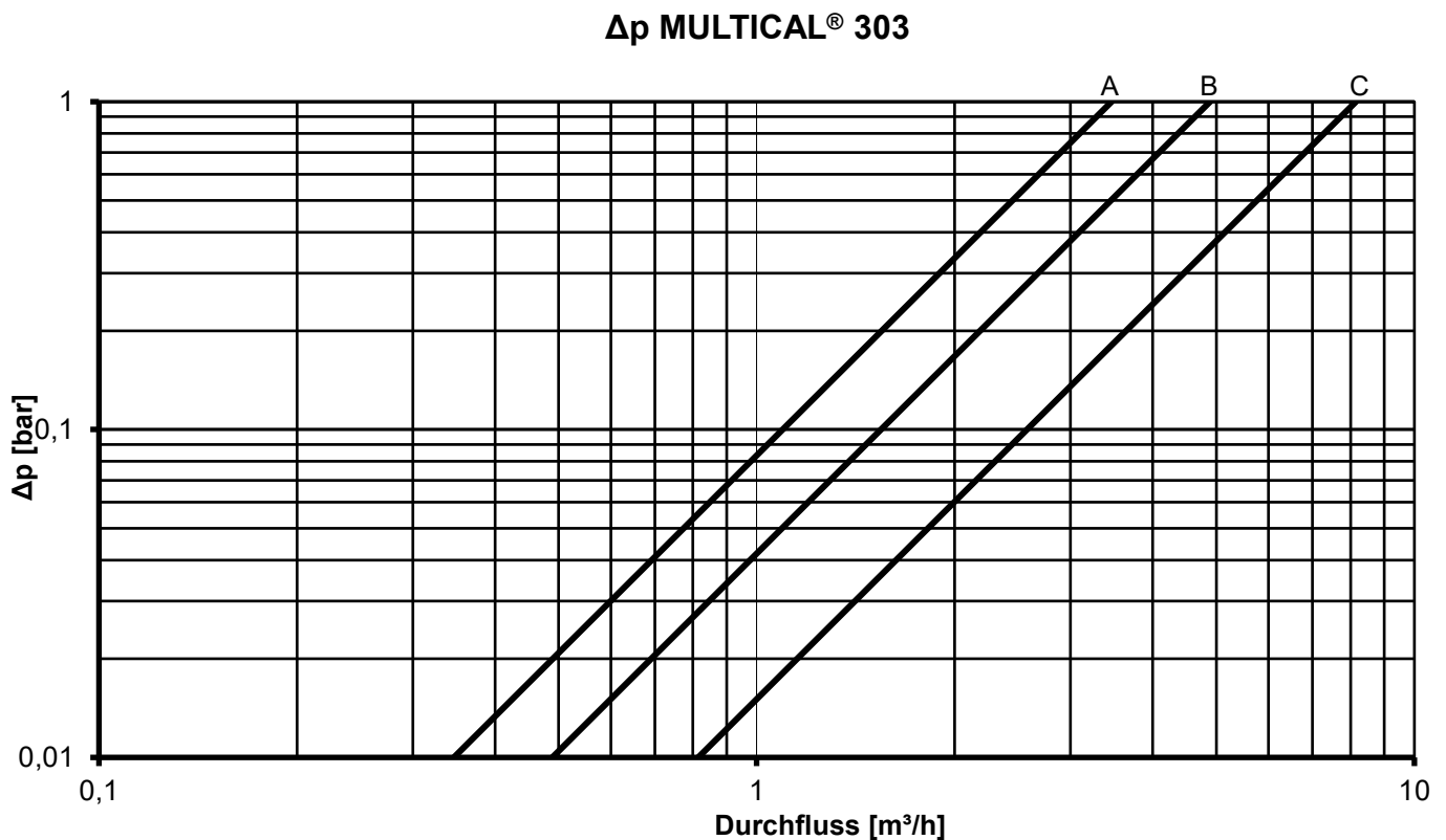
Diagramm 3: Druckverlustkurven
